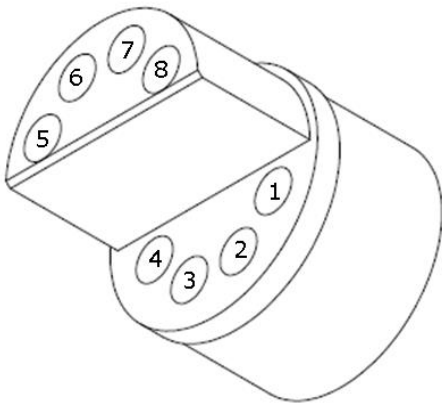
UW Receptacle Pin-out
